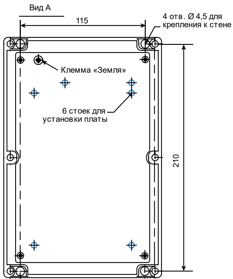
Рисунок 9.2 — Габаритные и установочные размеры изделия в корпусе 041
