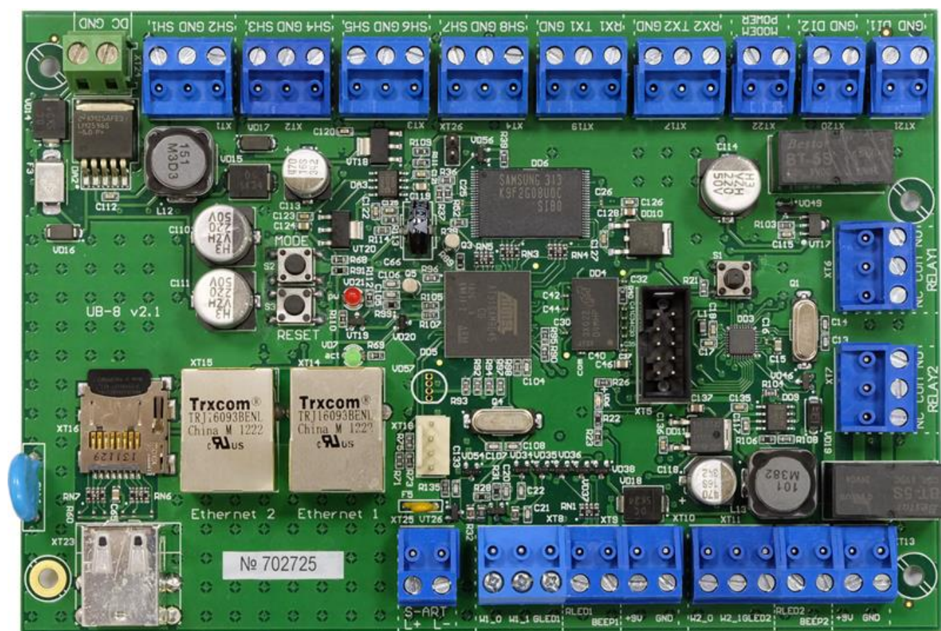
Рисунок 1.5 – Плата электроники контроллера «Борей». Внешний вид
