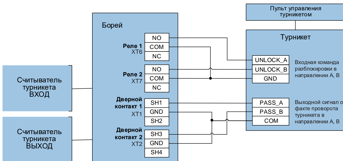
Рисунок 9.18 — Схема подключения турникета
