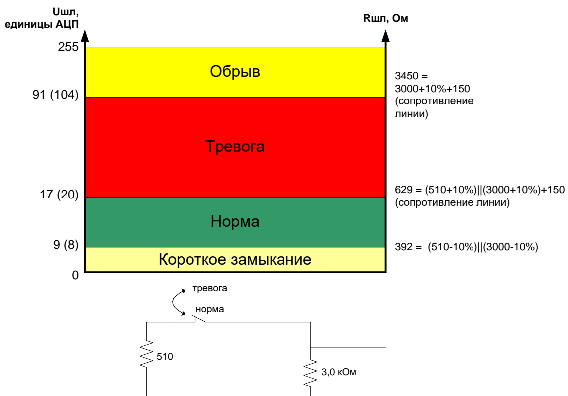
Рисунок 1.3 — Диаграмма порогов состояний при контроле цепи нагрузки
