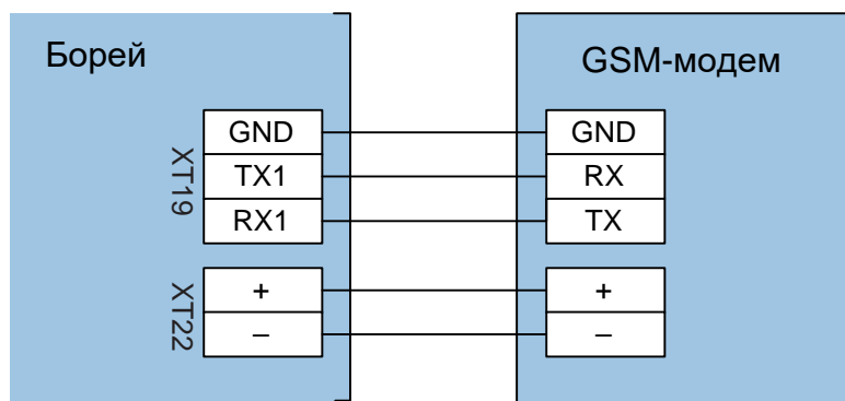
Рисунок 9.7 – Пример подключения GSM-модема по интерфейсу RS-232 с питанием от прибора
