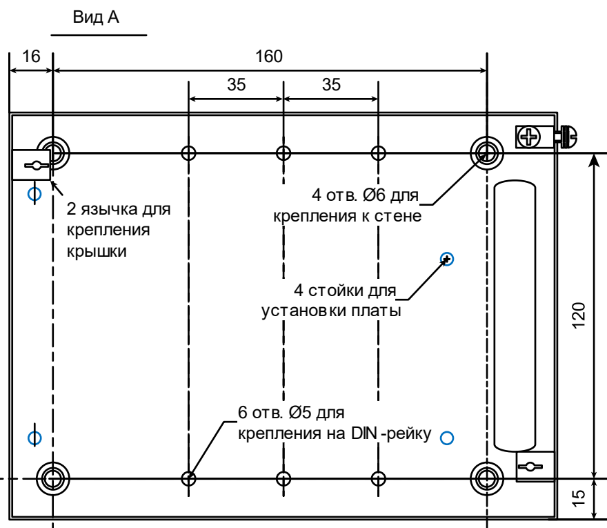
Рисунок 9.1 — Габаритные и установочные размеры изделия в корпусе 077
