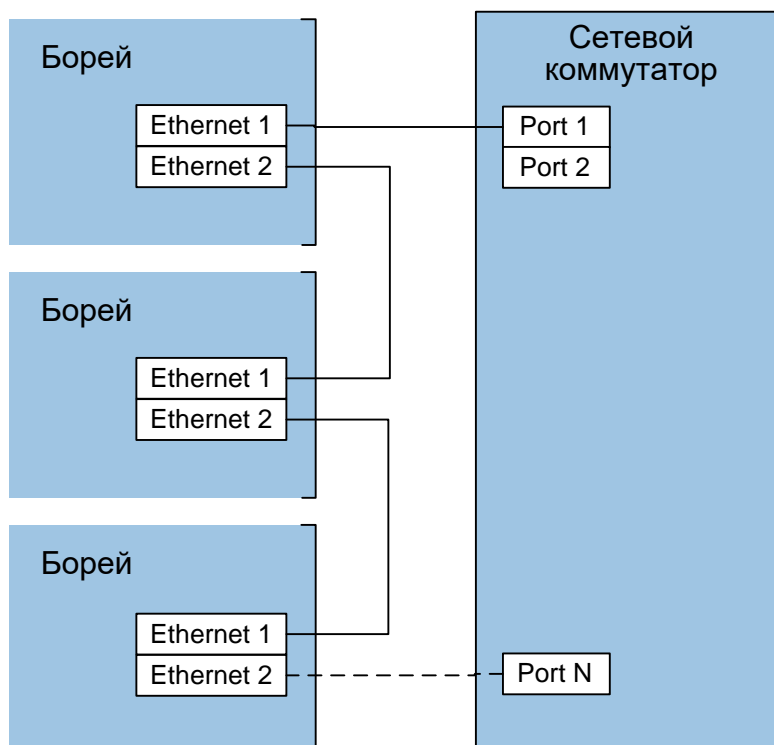
Рисунок 9.9 — Схема подключения приборов к сети Ethernet. «Коммутируемая IP-шина»
