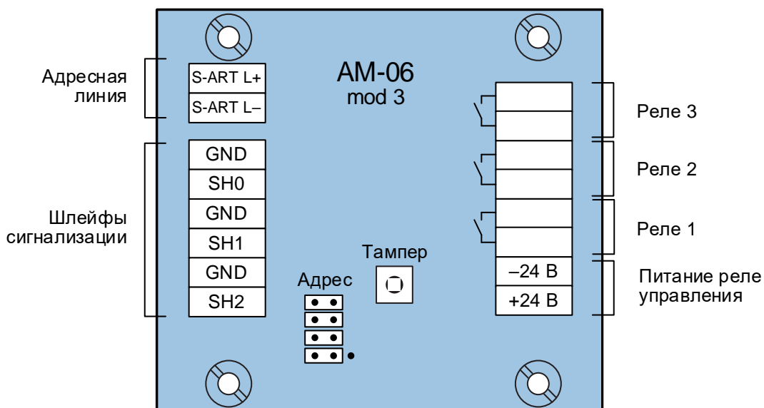
Рисунок 1.16 — Плата электроники «AM-06» в исполнении 3
