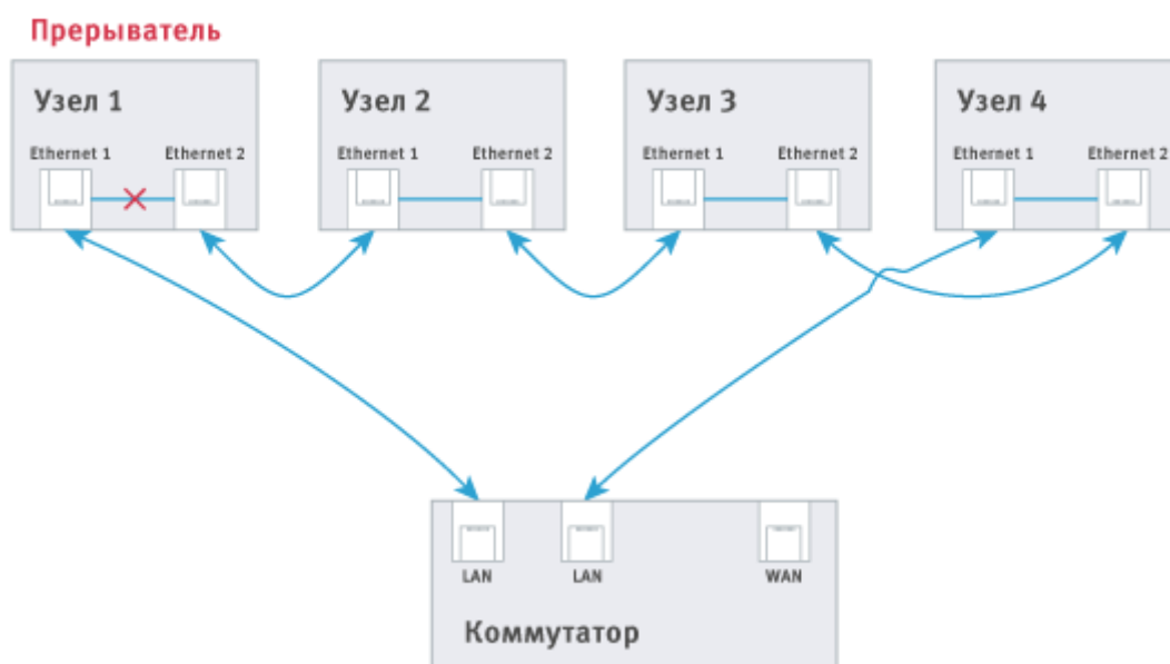
Рисунок 9.84 — Топология типа «кольцо» с прерывателем
