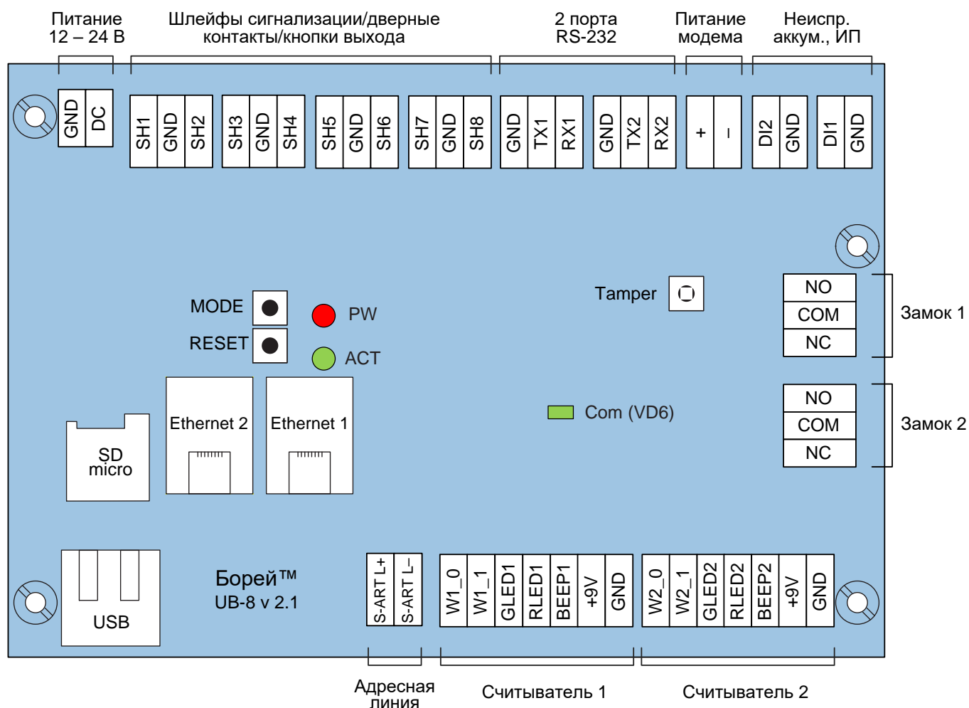
Рисунок 1.6 – Плата электроники контроллера «Борей». Схема расположения разъемов
