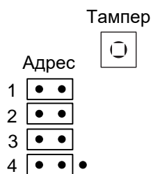
Рисунок 1.13 — Нумерация пар контактов для установки перемычек
