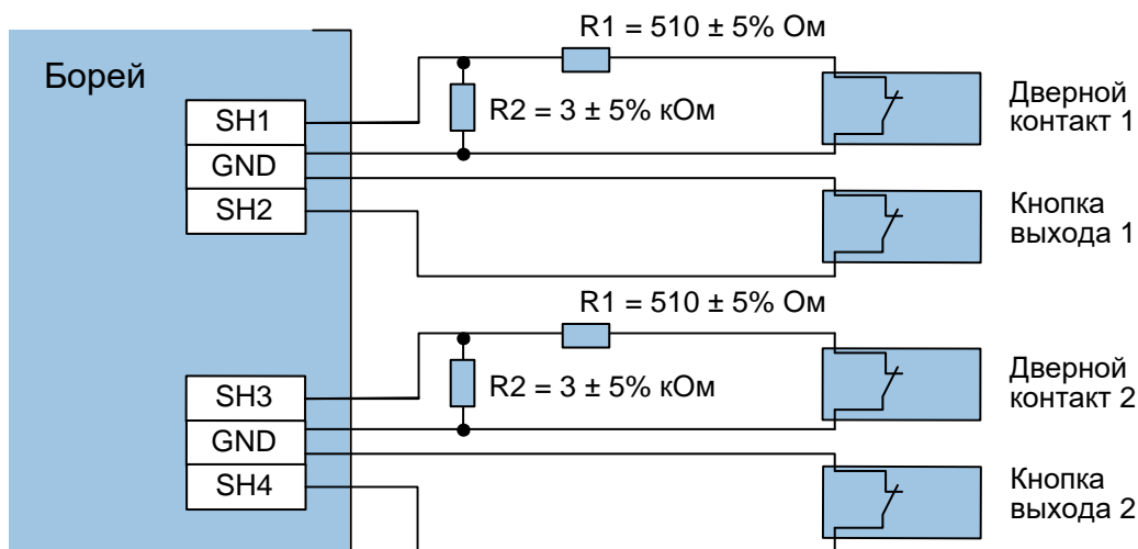
Рисунок 9.17 — Схема подключения дверных контактов и кнопок выхода
