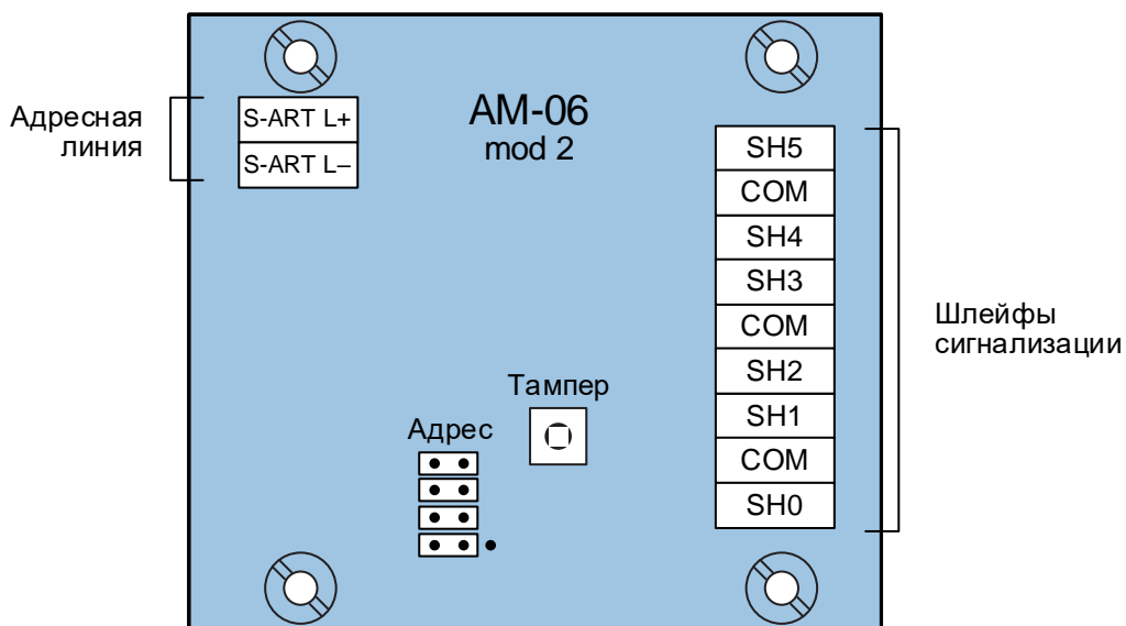
Рисунок 1.15 — Плата электроники «AM-06» в исполнении 2
