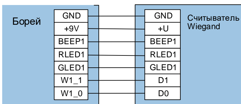
Рисунок 9.13 — Схема подключения считывателя с интерфейсом Wiegand
