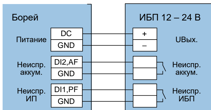
Рисунок 9.6 – Схема подключения источника бесперебойного питания (ИБП)
