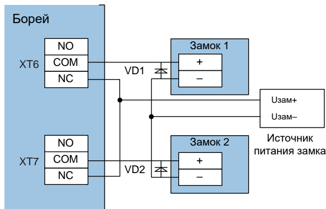
Рисунок 9.16 — Схема подключения замкового устройства
