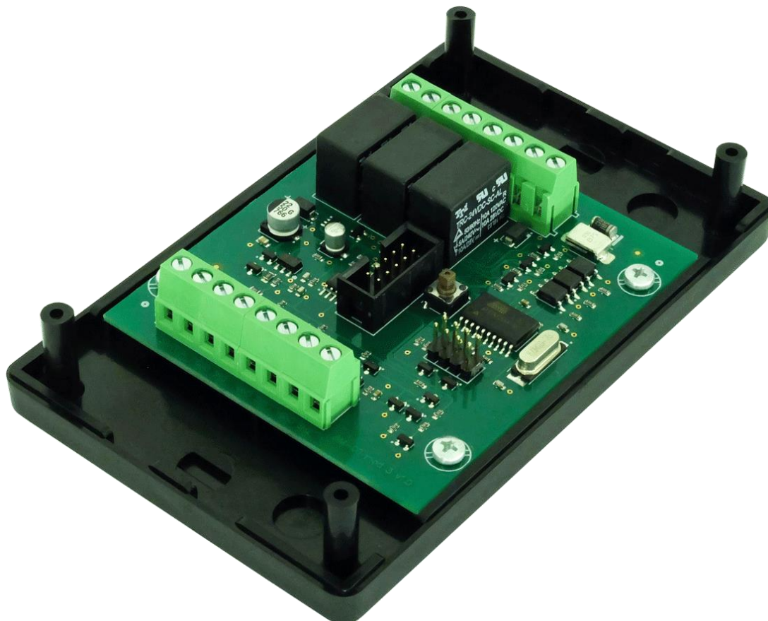
Рисунок 1.14 — Общий вид «АМ-06»
