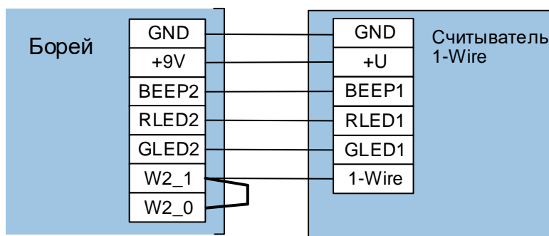
Рисунок 9.14 — Схема подключения считывателя с интерфейсом 1-Wire
