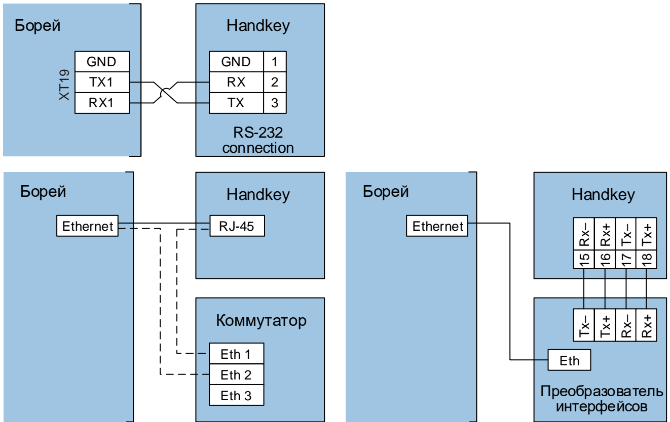
Рисунок 9.21 — Схема подключения Handkey-II посредством интерфейсов RS-232, Ethernet и RS-422
