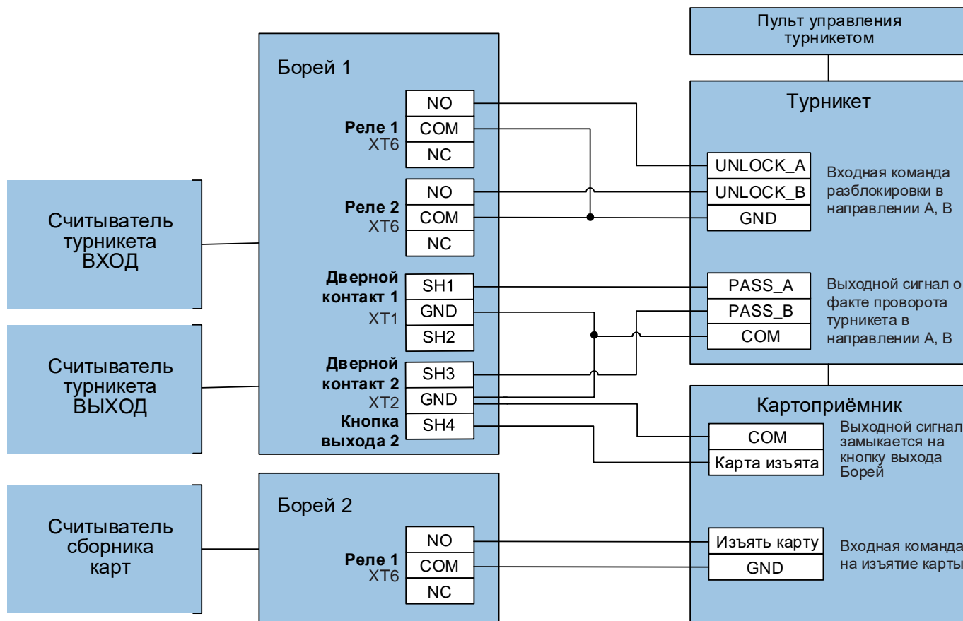
Рисунок 9.19 — Схема подключения картоприёмника
