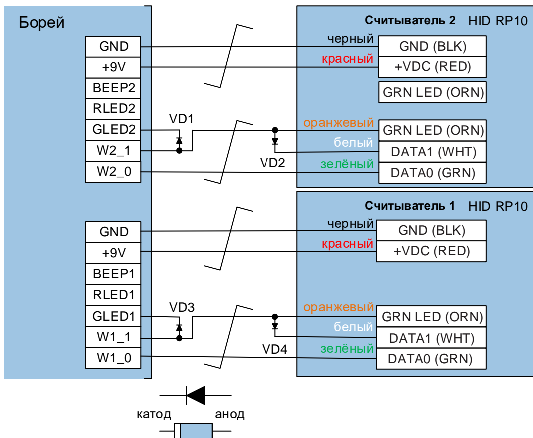
Рисунок 9.15 — Схема подключения считывателя HID RP10 (с использованием четырехпроводного кабеля)
