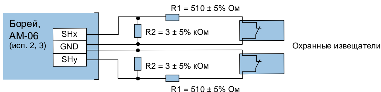
Рисунок 9.12 – Схема подключения ШС с датчиками типа «сухой контакт» к контроллеру «Борей» и расширителям «АМ-06» в исполнениях 2 и 3
