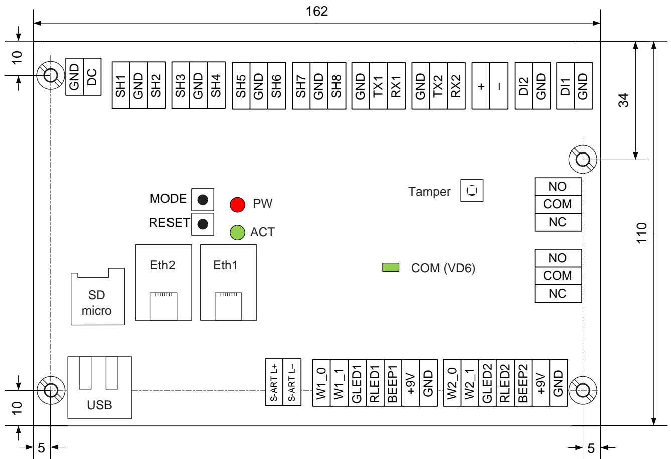
Рисунок 9.4 — Габаритные и установочные размеры платы «Борей»
