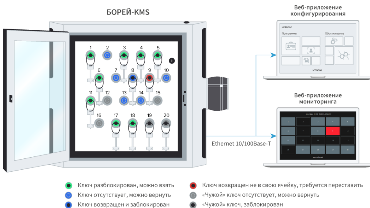
Рисунок 1.9 — Схема изделия и режимы индикации
