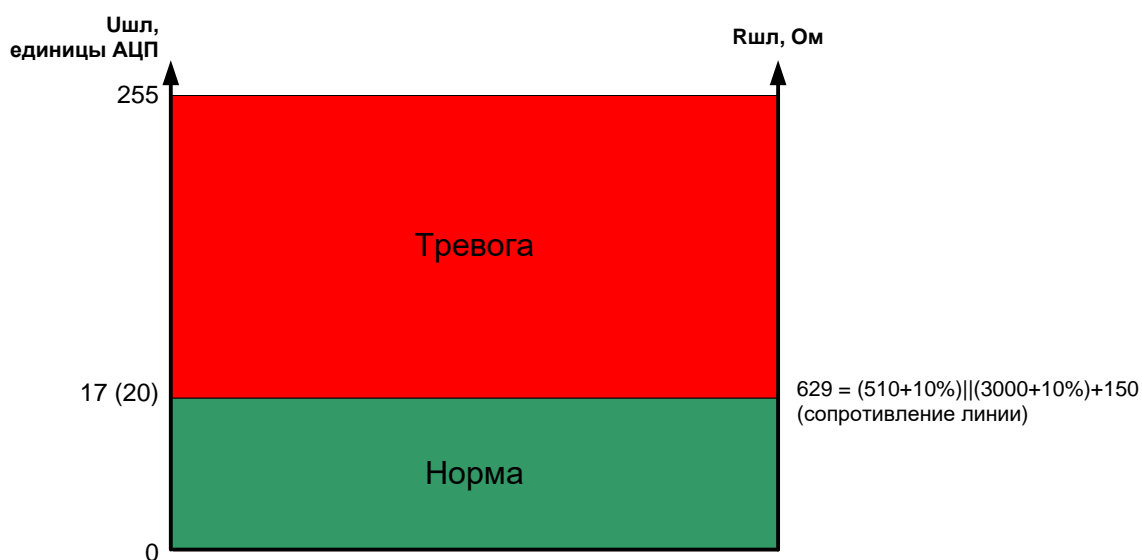
Рисунок 1.4 — Диаграмма порогов состояний без контроля цепи нагрузки
