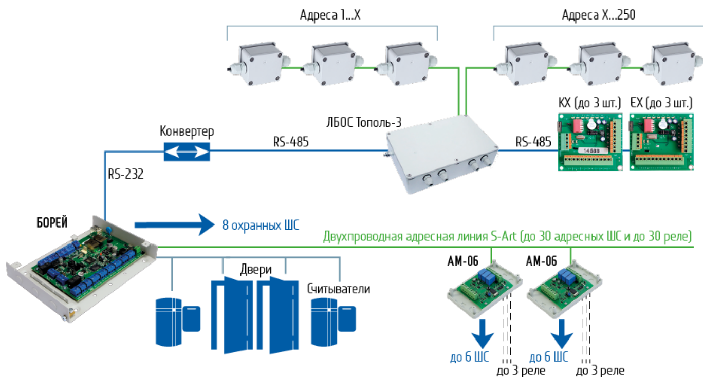
Рисунок 1.7 — Общая схема подключения комплекса Тополь-3
