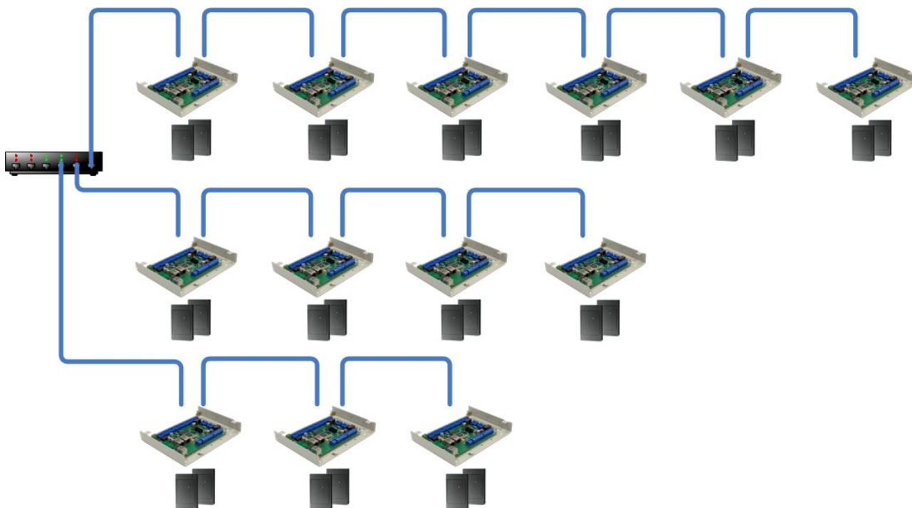
Рисунок 9.10 — Схема подключения приборов к сети Ethernet. Произвольная архитектура
