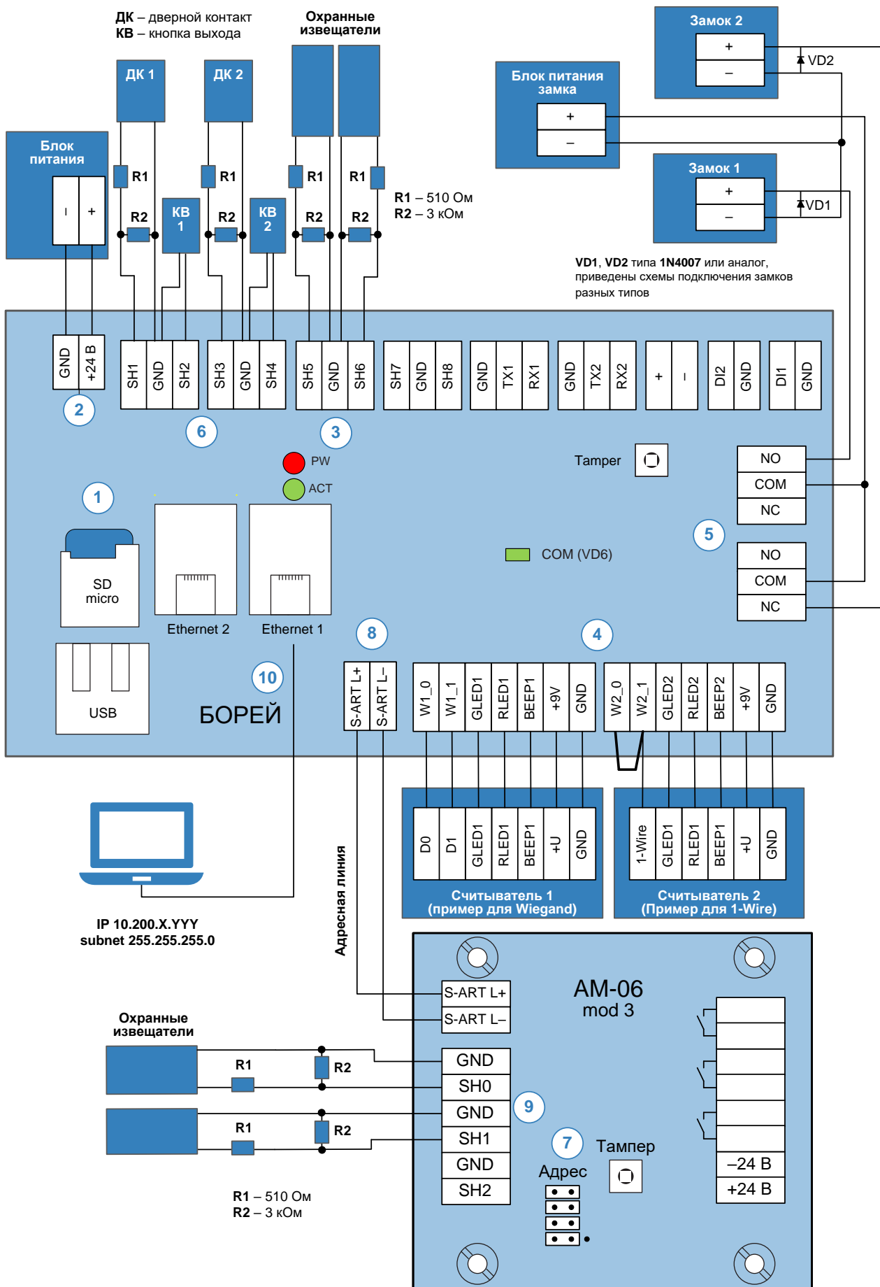
Рисунок 2.1 — Схема подключения прибора «Борей»
