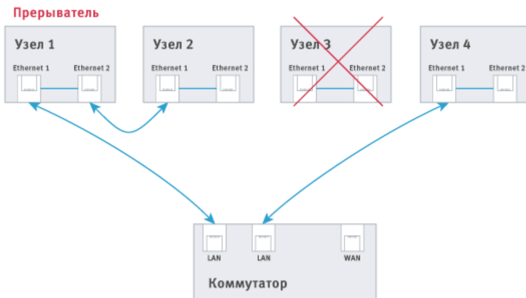
Рисунок 9.85 — Топология типа «кольцо» с прерывателем. Потеря связи с узлом 3.
