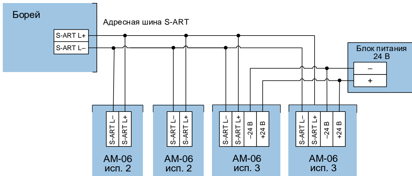
Рисунок 9.11 — Схема подключения расширителей «АМ-06» к адресной линии
