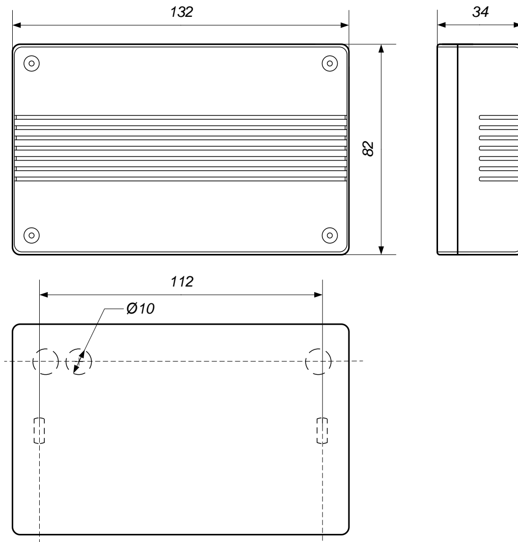
Рисунок 9.5 — Габаритные размеры «АМ-06» в корпусе 115
