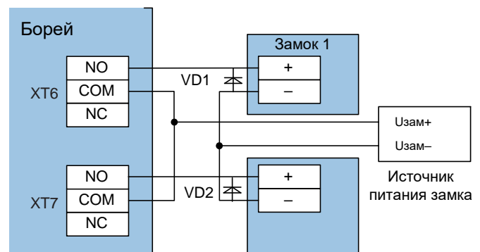
Рисунок 9.16 — Схема подключения замкового устройства
