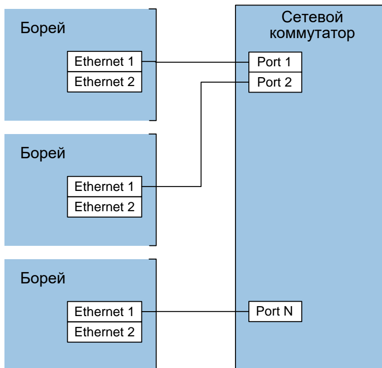
Рисунок 9.8 – Схема подключения приборов к сети Ethernet. Классический вариант
